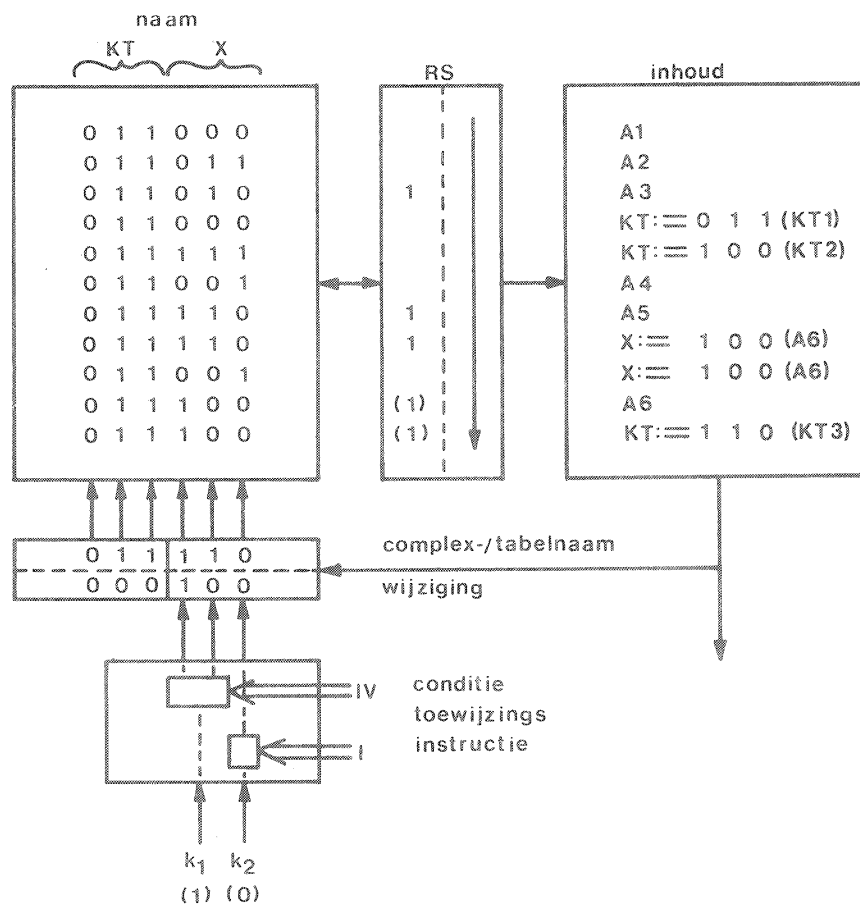
Fig.3.8.geheugenvulling met programma van Fig.3.6.
