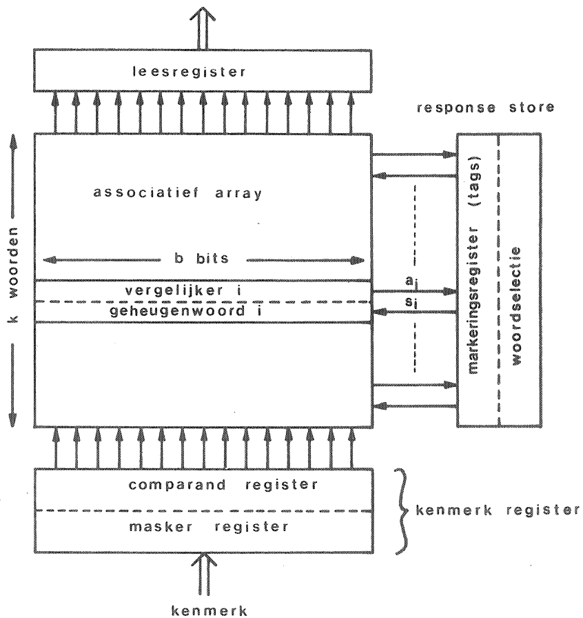
fig. 1.3 Blokschema associatief geheugen.
