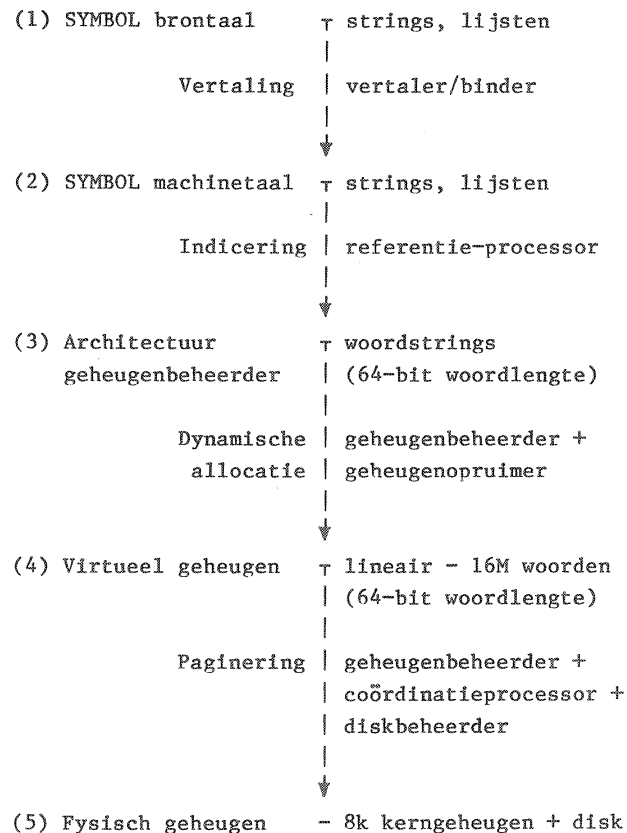
Fig. 2 - SYMBOL geheugenniveaus
