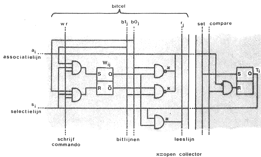
fig. 2.1. Bitslice j van het kenmerkregister.
