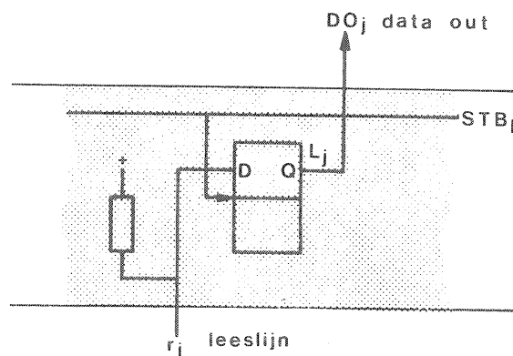
fig.2.3. Bitslice van het leesregister.
