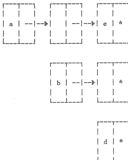
Figuur 2. Representatie van een LISP lijst.
