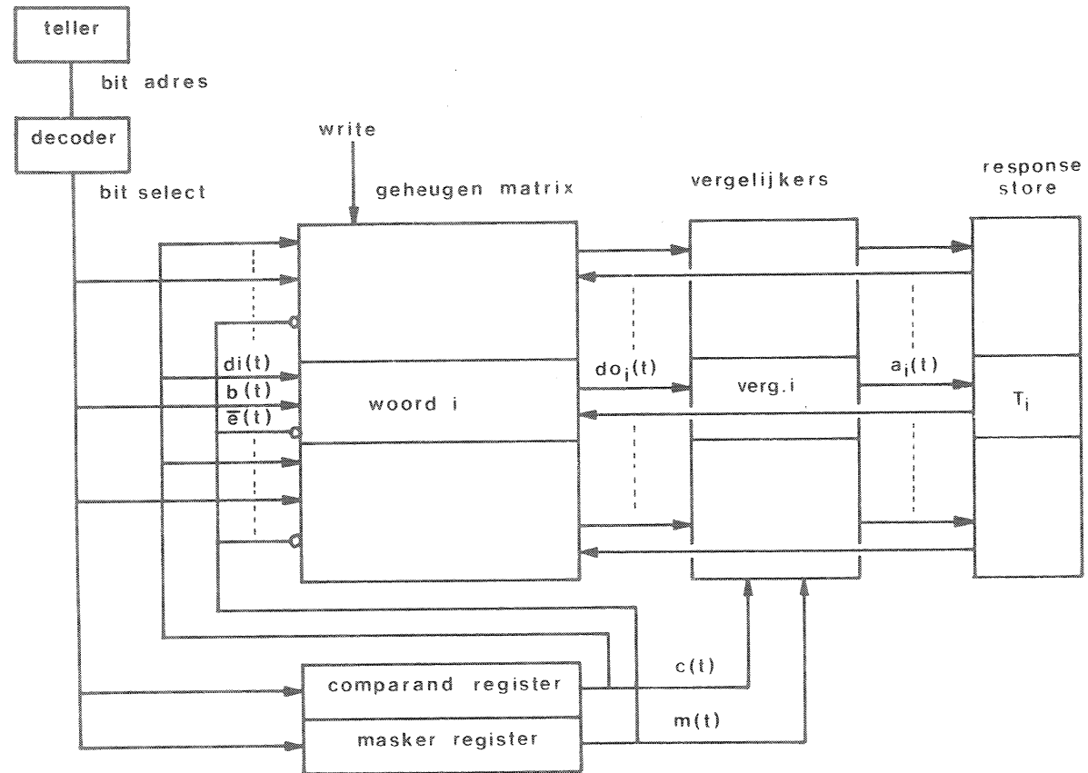
fig. 3.2. Bit serieel associatief geheugen.
