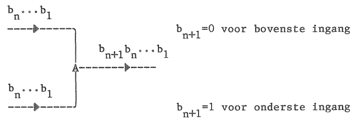
Fig. 11. Arbiter.
