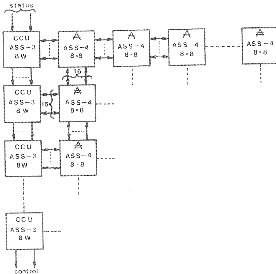
fig.4.1. Associatief geheugen m.b.v. ASS-3 (CCU) en ASS-4(A).
