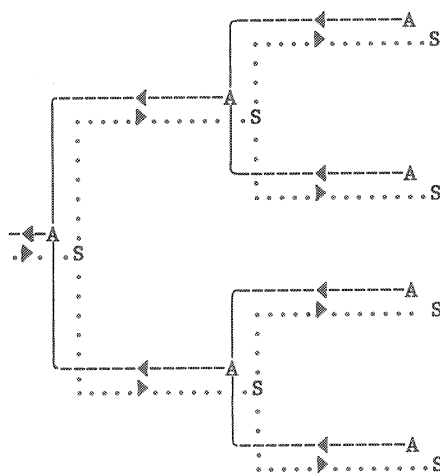
Fig. 13. Adressering met arbiter/selector paren.
