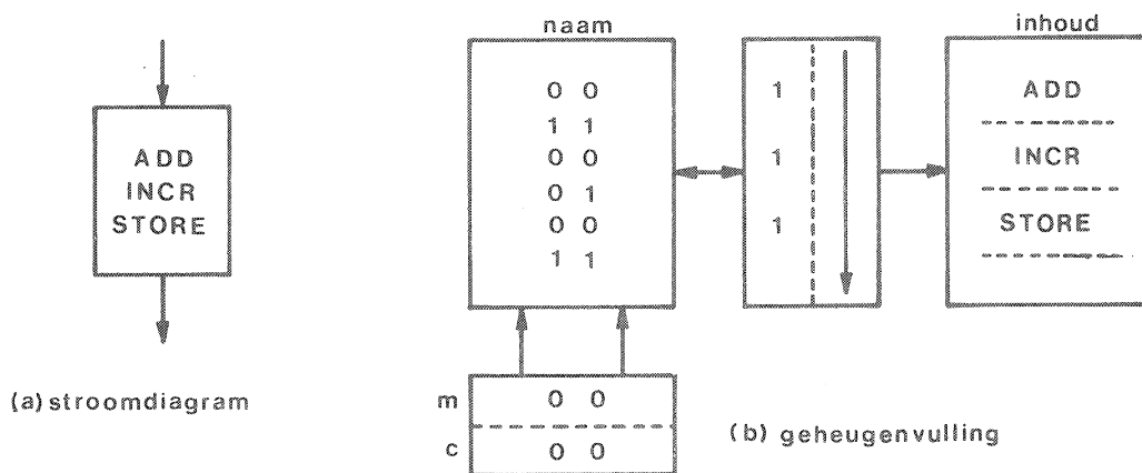
Fig.3.3. implementatie lineaire tak
