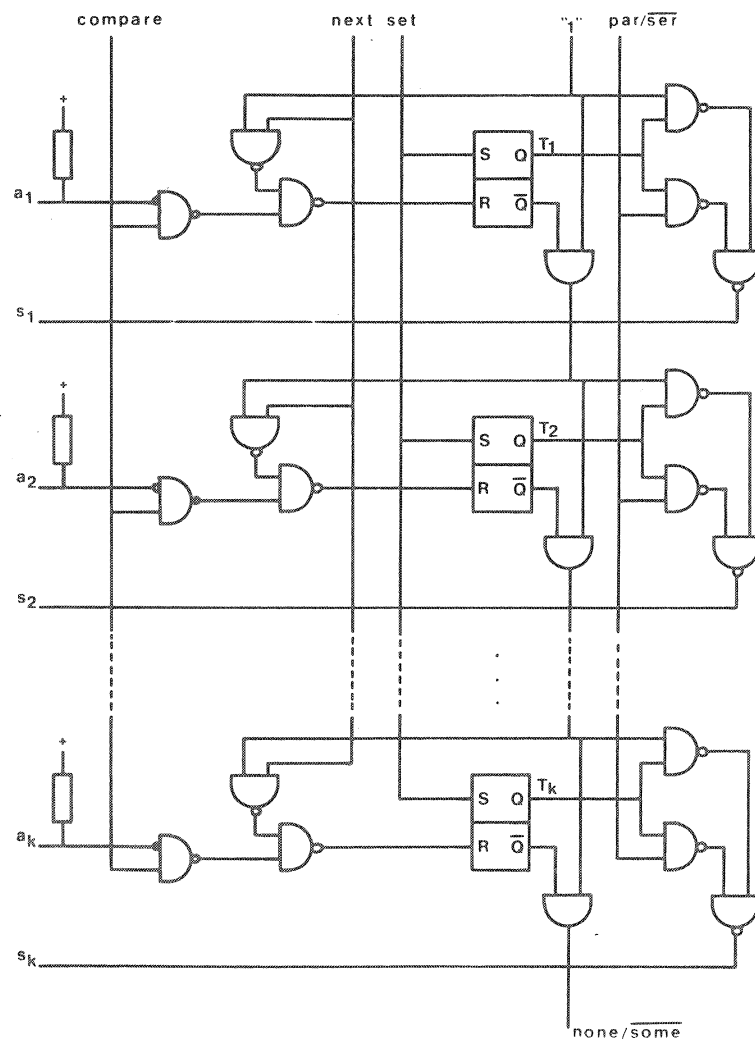
Fig.2.4. Response store.
