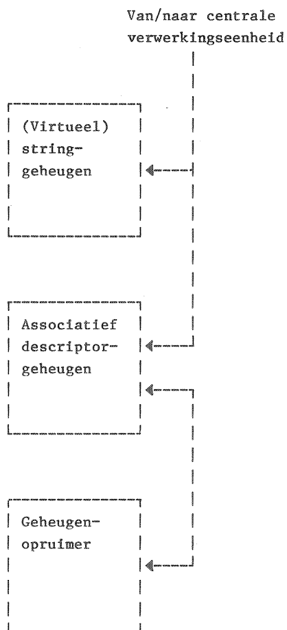
Fig. 3 - Blokdiagram string-geheugen
