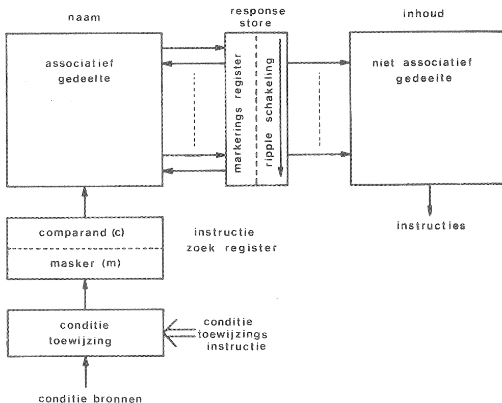
Fig.3.2. structuur van een associatief werkgeheugen met betrekking tot het ophalen van instructies
