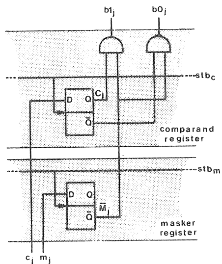
fig. 2.1. Bitslice j van het kenmerkregister.
