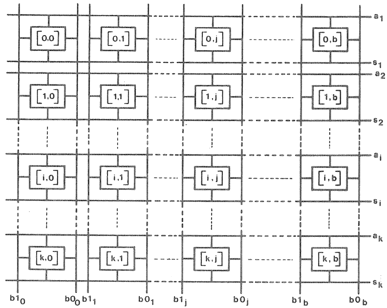
fig. 4.2. Organisatie van het associatief array m.b.v. ASS-4.
