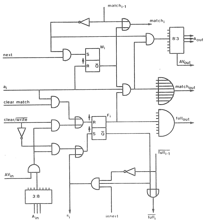
fig.4.6. besturing van één woord.
