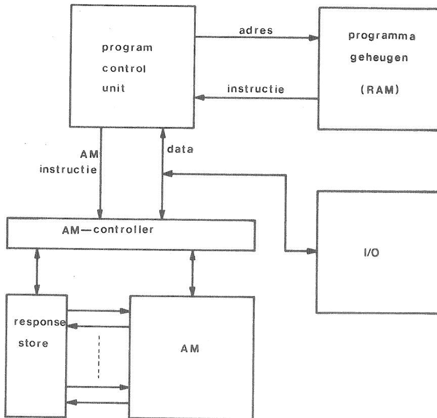
Fig.2.1. architectuur van een machine met een associatief datageheugen
