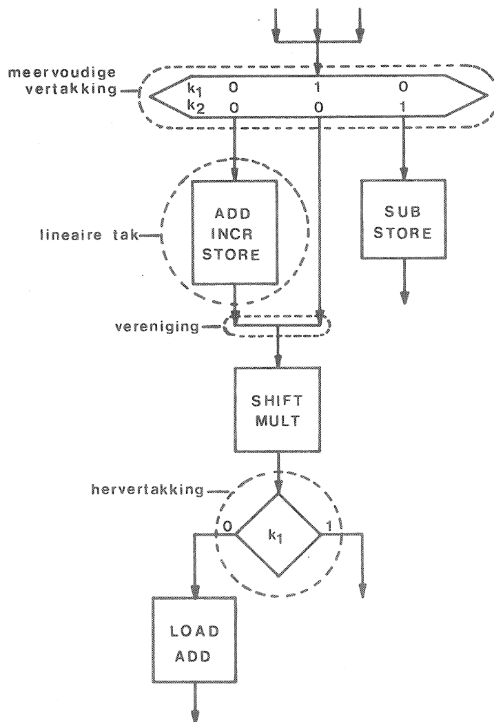
Fig.3.1. programmastructuur-elementen
