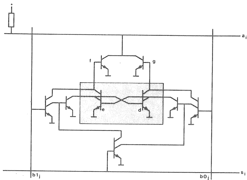
fig. 4.4. Geheugencel in 1^2L .
