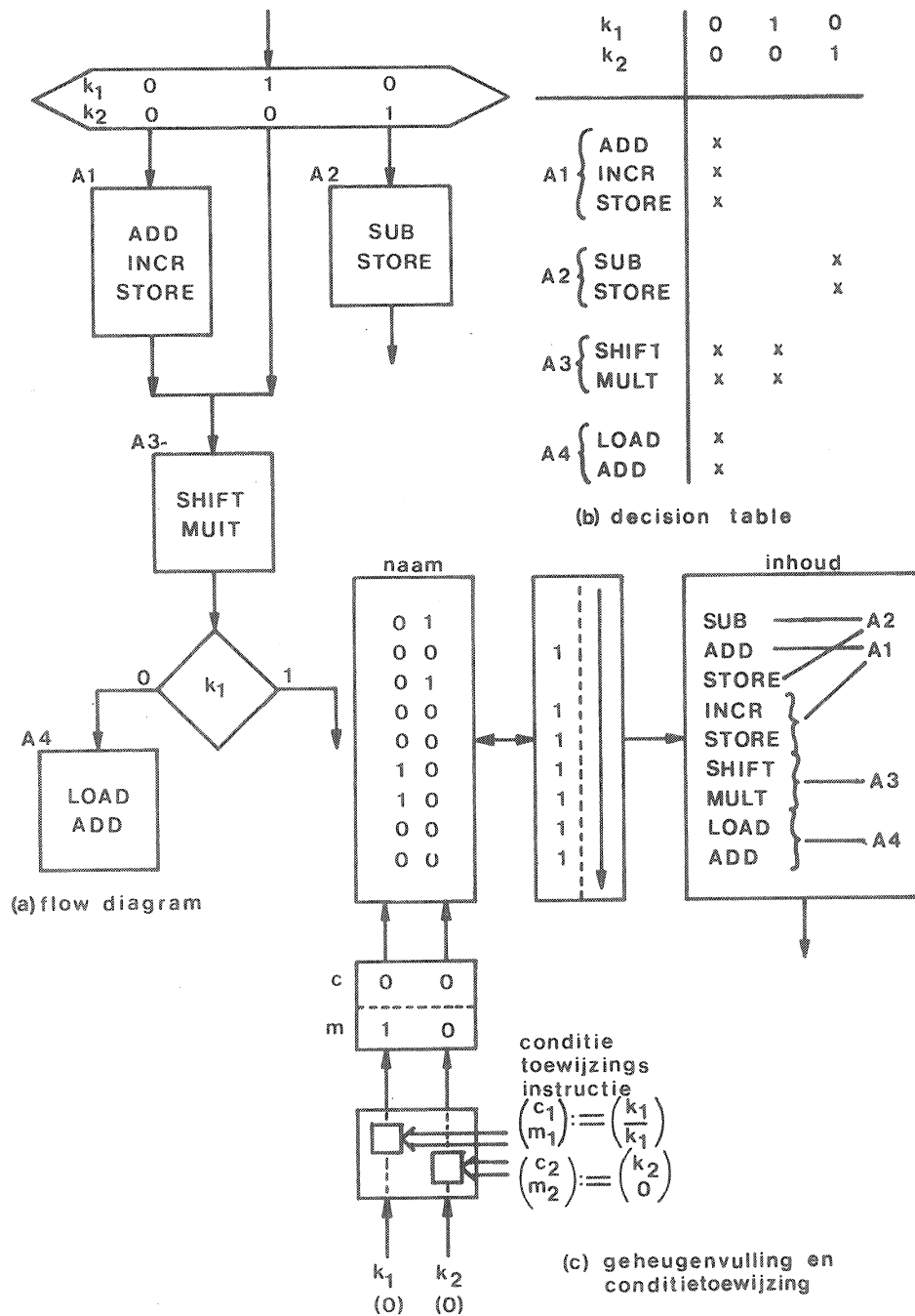
Fig.3.5. implementatie van vereniging ( met hervertakking )
