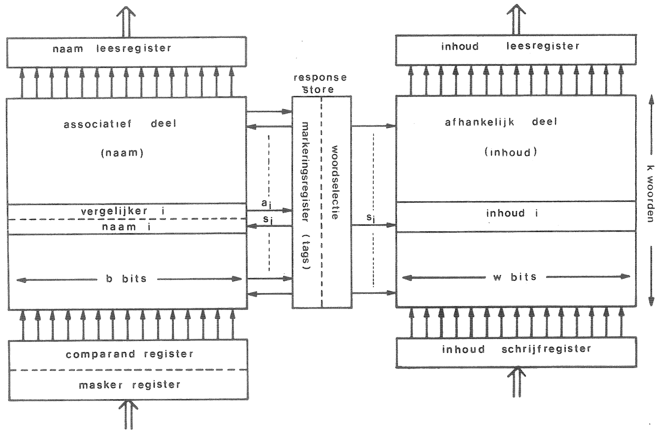
fig. 3.1. Partieel associatief geheugen.
