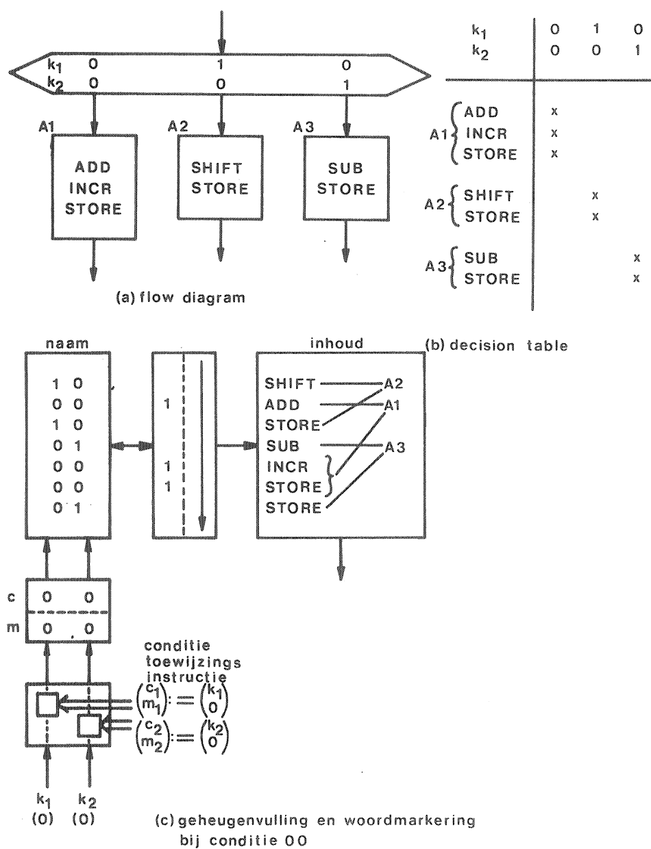
Fig.3.4. implementatie van vertakking
